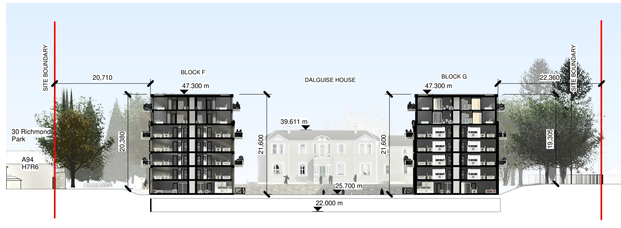
Section D-D 1 : 500
